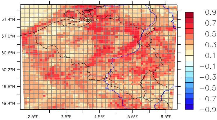
MAR-MIRhisto (1976-2005)
