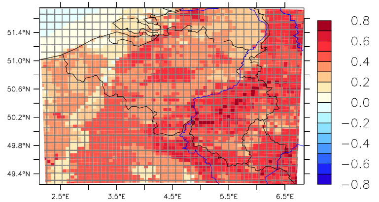
MAR-NORhisto (1976-2005)
