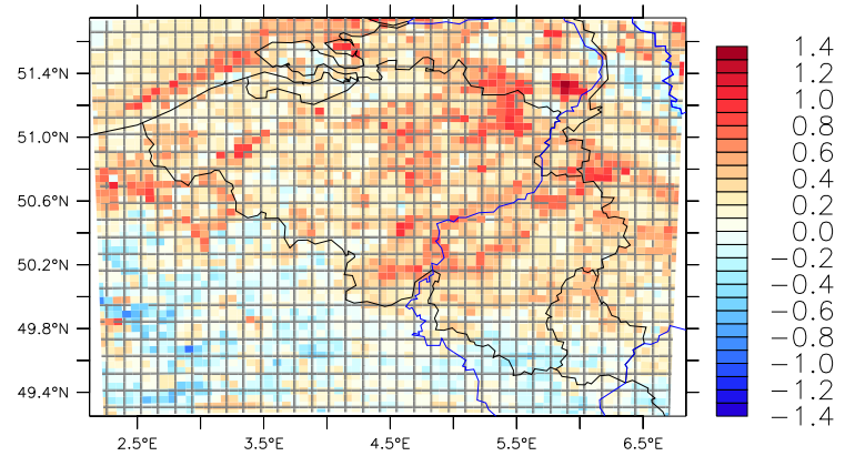
MAR-NORhisto (1976-2005)
